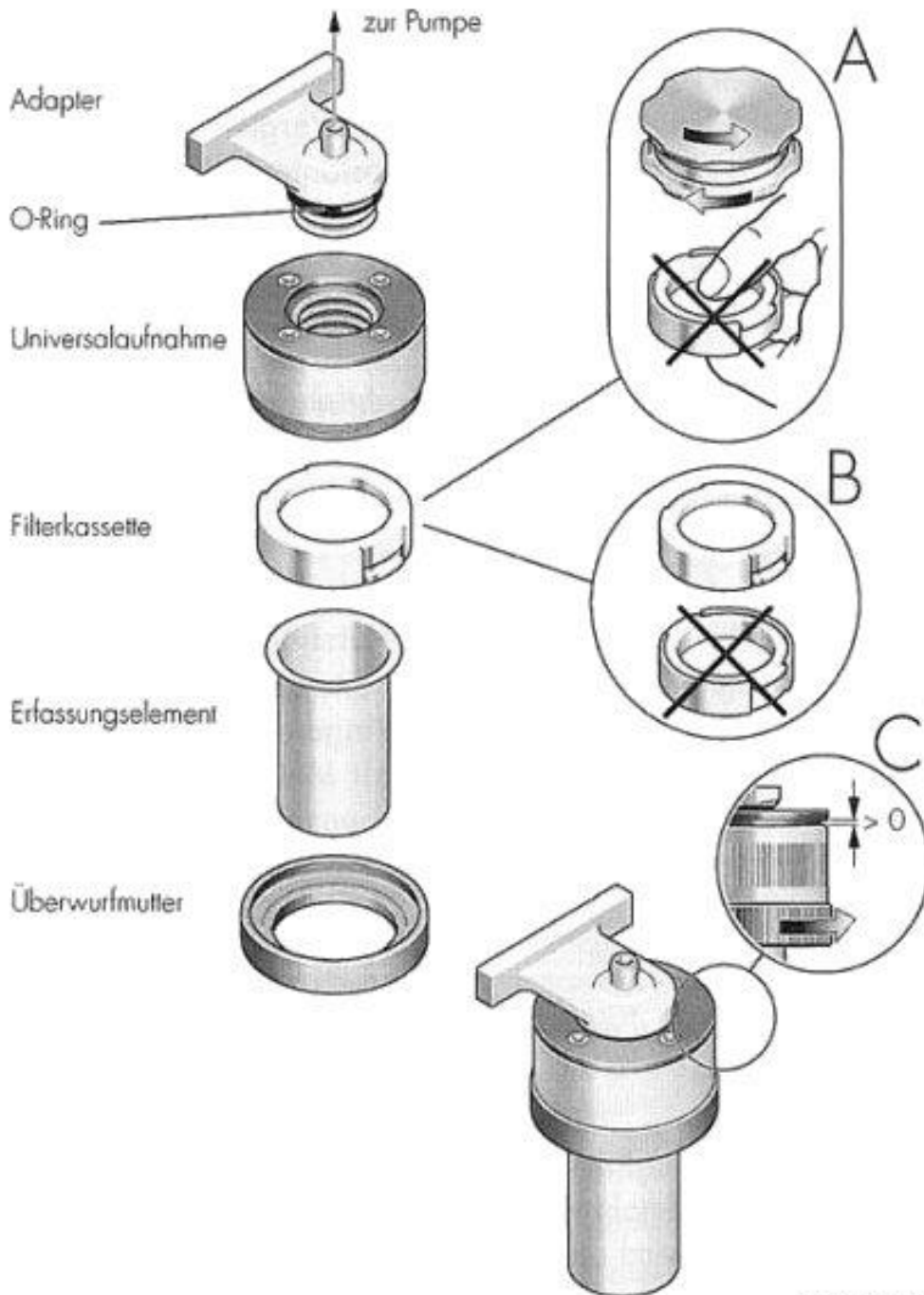
PGP-System - FAP für Faser-Probenahme (Probenahmenvolumen 2.0 l/min)
